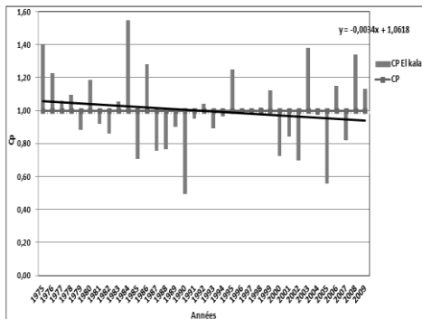
Figure 12 : Evolution des anomalies pluviométriques dans la station d'El kala
