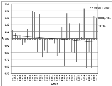
Figure 15 : Evolution des anomalies pluviométriques dans la station des Salines
